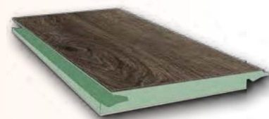
Schwimmende Verlegung auch in Feuchträumen Installation flottante, même dans les pièces humides
